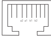
Belegung der externen S0s
