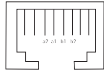
Belegung der internen S0s
